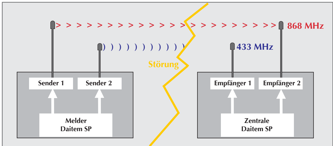
Schematische Darstellung der Funk-Übertragung
