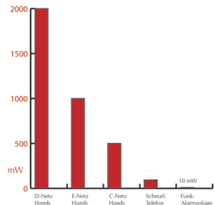
Vergleich der maximalen Sendeleistung
